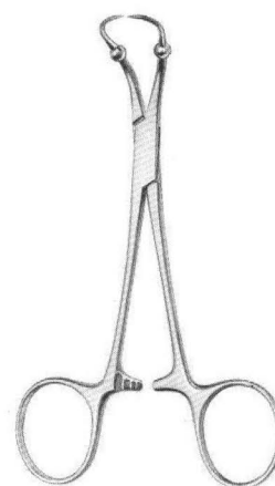
Roeder 07-687-13 13 cm 07-687-15 15 cm
